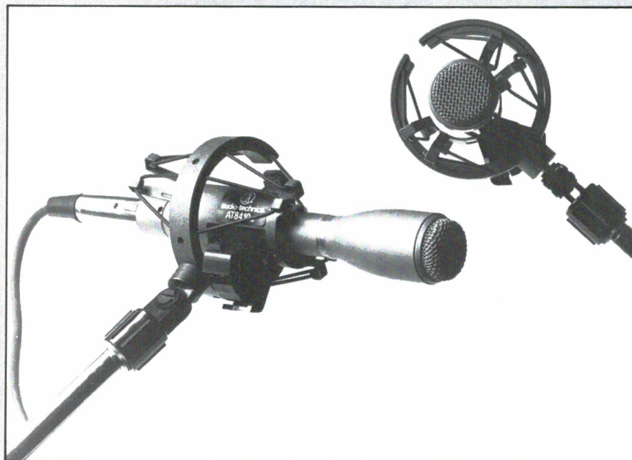
Foto 2. Vloertrillingen die via het microfoonstatief tot de microfoon doordringen zijn funest voor de opname. Gebruik in zo'n geval een verende opstelling, zoals de hier afgebeelde speciale shock mount.
